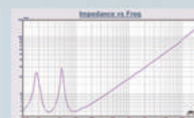
SW-V12 阻抗曲线
