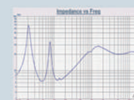
KS-710 阻抗曲线
