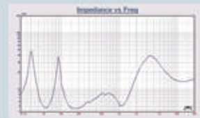
PL-12 阻抗曲线
